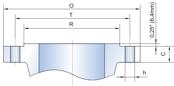
CLASS 600-2500 RF
