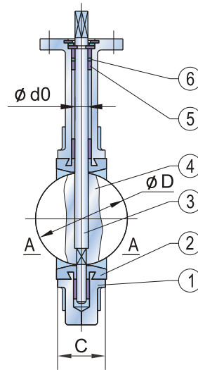
A-A SECTION
