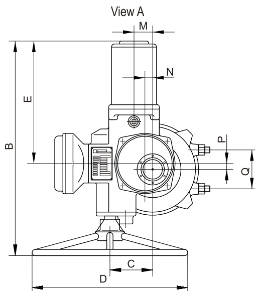
Type 9034/4027
