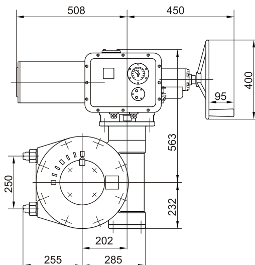
Type 9034/4027
