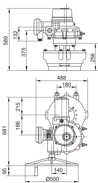
Type 802. 1000-0. 2
