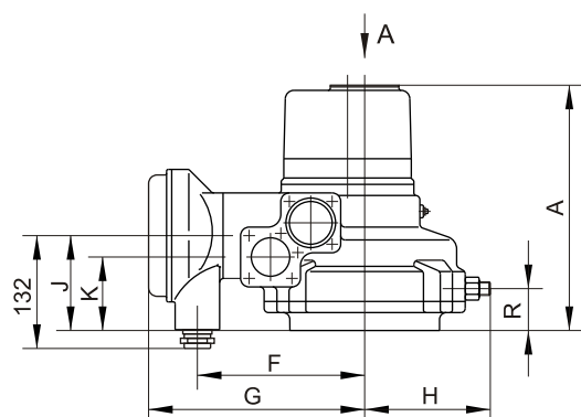
Type 802. 1000-0. 2
